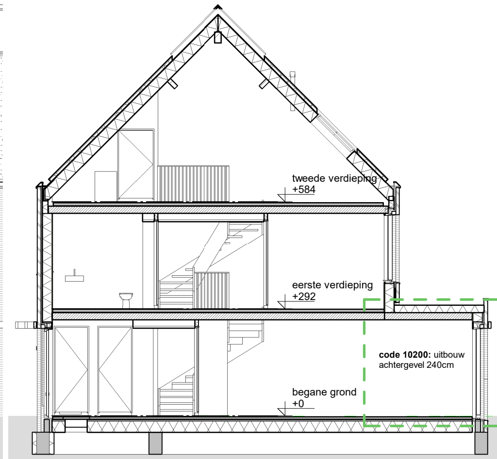
langsdoorsnede
