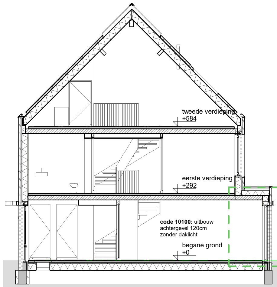
langsdoorsnede
