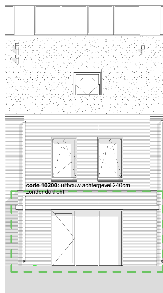
achtergevel
