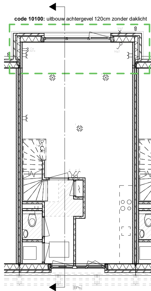
Ba optie 1 00 begane grond
